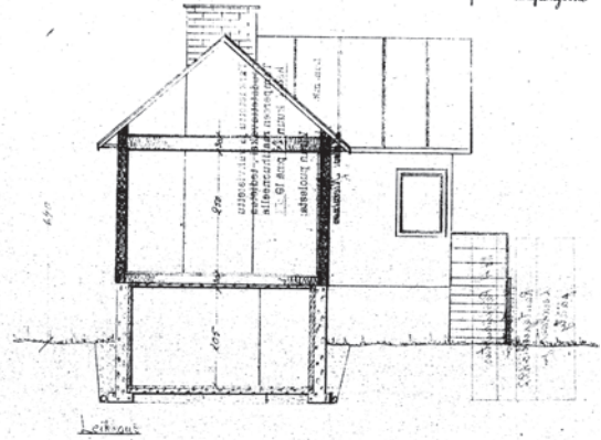
Leikkaus.
