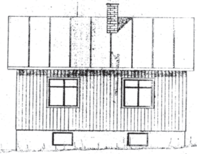
Julkisivu itään.
